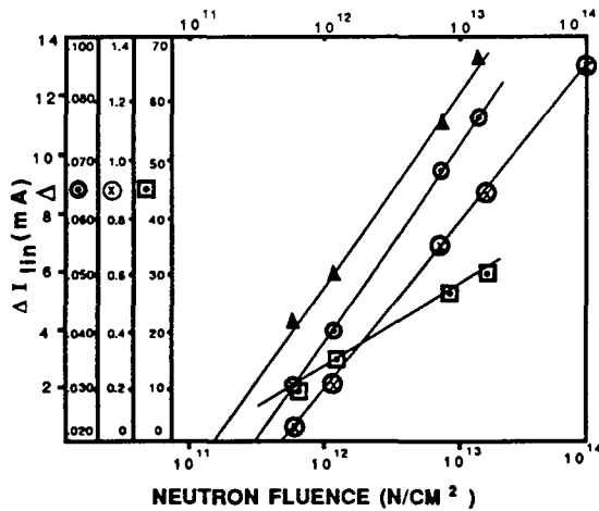
Fig 6: Decrease in the photodiode linearity vs neutron fluence. □ p-p+ epitaxial, 25 ohm-cm, I_{lino} = 75 mA ▲ 400 ohm-cm n-type (UDT PIN 1223), I_{lino} = 14 mA ● 400 ohm-cm n-type (UDT FIL C10D), I_{lino} = 80 \mu A ⊙ 100 ohm-cm n-type (UDT FIL 6230), I_{lino} = 1.5 mA
